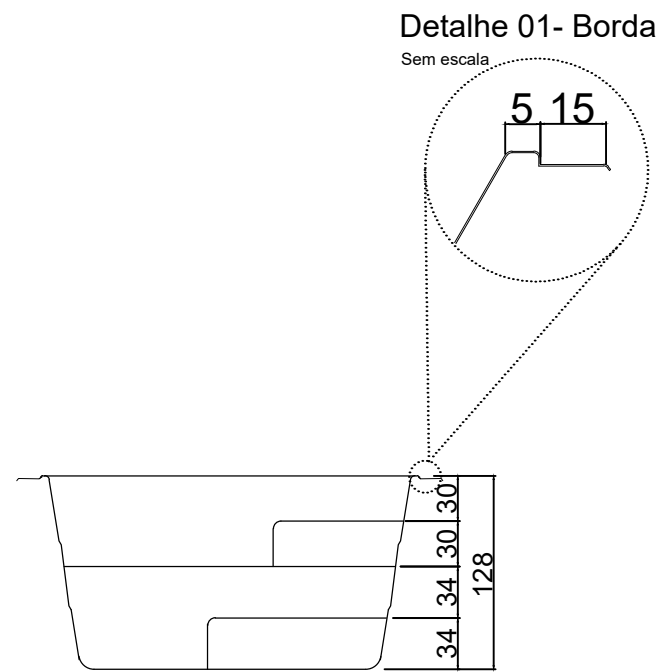
CORTE B Esc: 1:50
