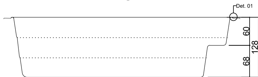
CORTE A Esc: 1:50
